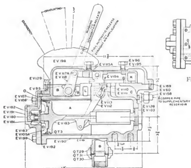
Fig. 2579. Longitudinal Section.
